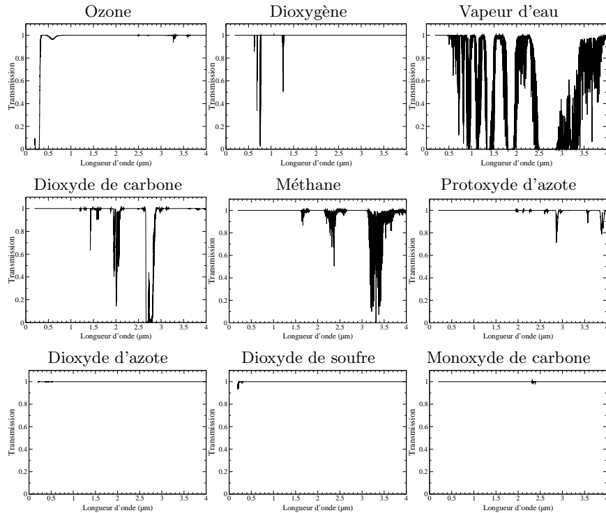
Figure 5.14 – Transmissions atmosphériques dans le domaine solaire pour le dioxygène et différents gaz traces.
