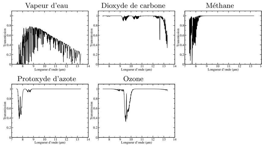
Figure 5.15 – Transmissions atmosphériques dans la fenêtre du domaine infrarouge pour différents gaz traces. Un profil tropical typique a été utilisé.
