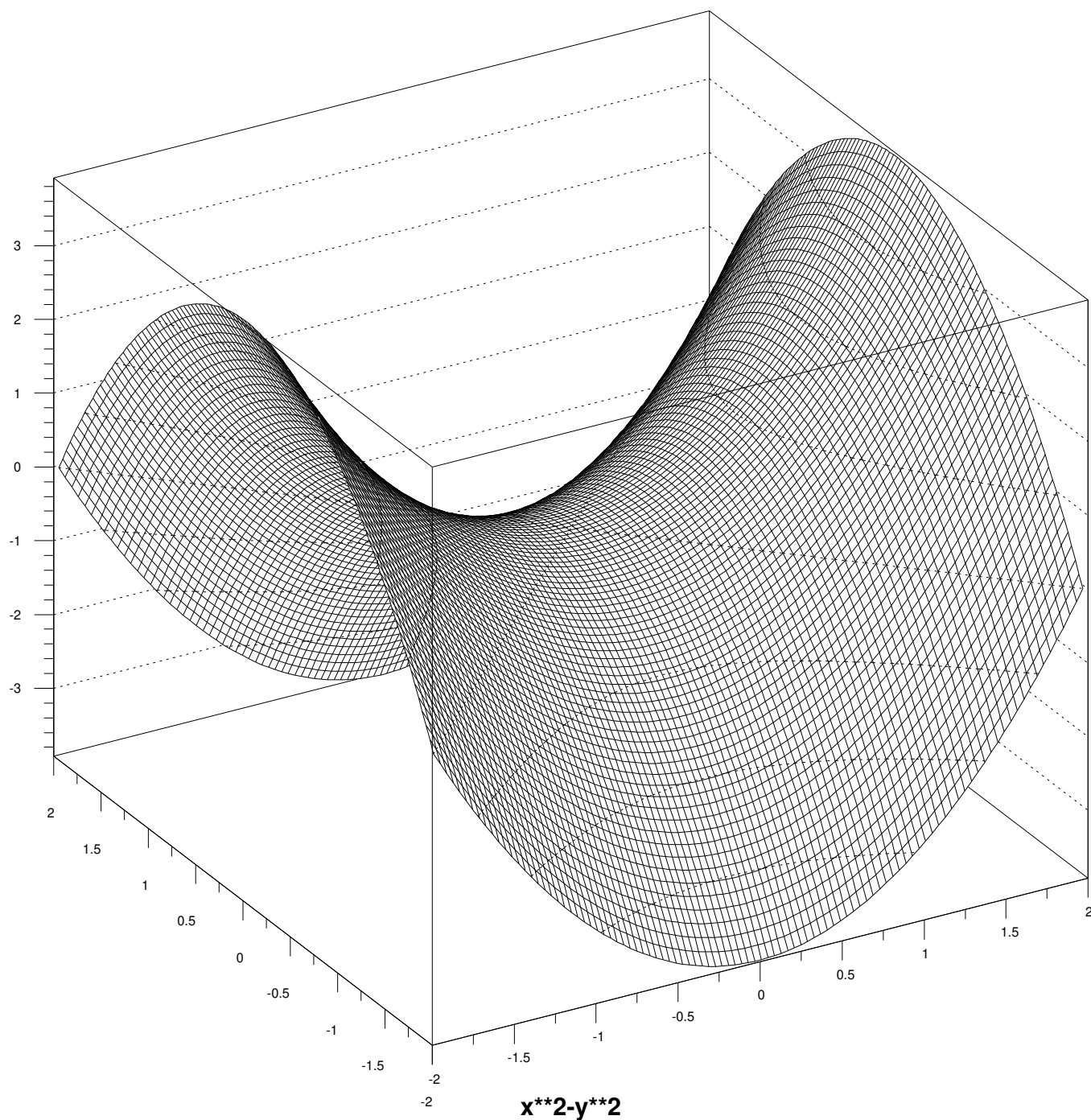
FIGURE 1 – Partie réelle de z^2 ( = x^2 - y^2 )
