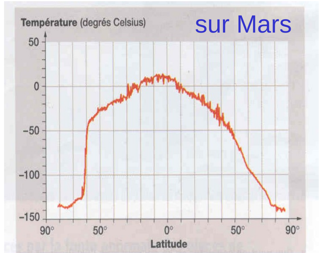
Température sur Mars (en degré Celsius) en fonction de la latitude.
