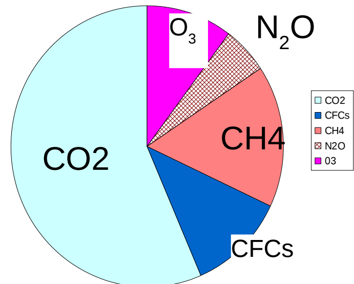
Effet de serre du aux activité humaine
