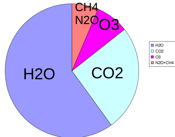
Contribution à l'effet de serre
