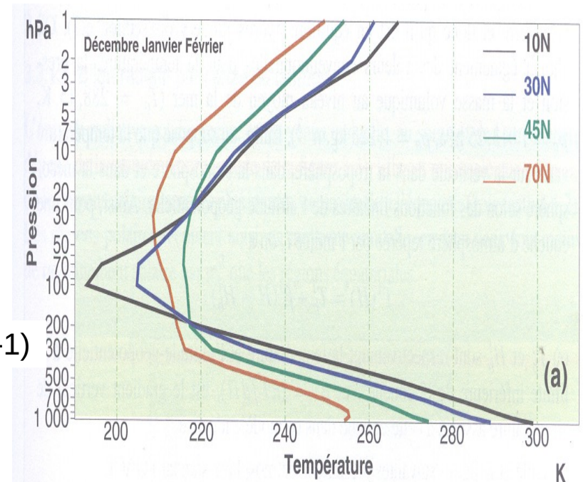
Profil vertical de température
