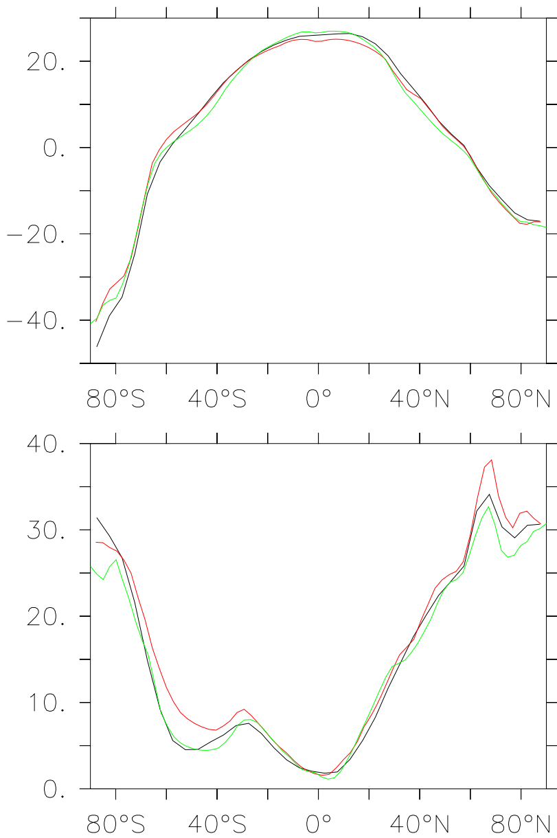
Figure 5: Moyenne zonale de la température (°C) de l'air près de la surface, sur la période 1960-1989, observée (en noir), et simulée par les modèle du CNRM (en rouge) et de l'IPSL (en vert). En haut, moyenne annuelle. En bas, amplitude du cycle saisonnier. Les observations utilisées sont celles compilées par le Climatic Research Unit (CRU) aux Royaumeis Unis [Jones et Moberg, 2003]
